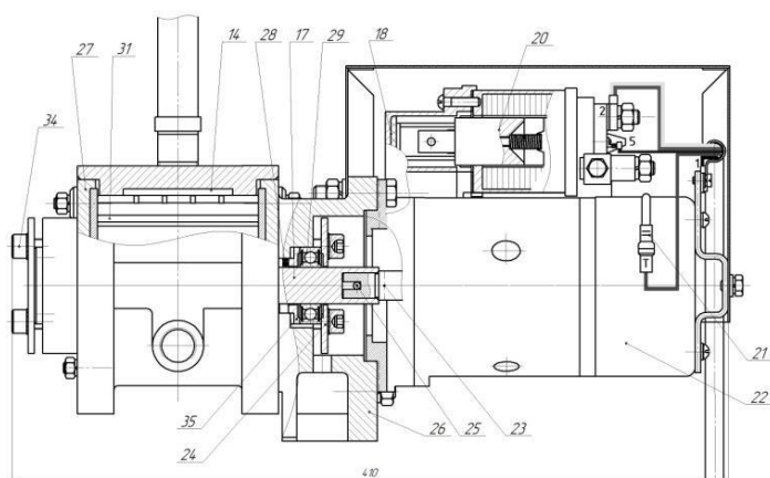
Рис. 3 Насос вакуумный электрический с системой управления
