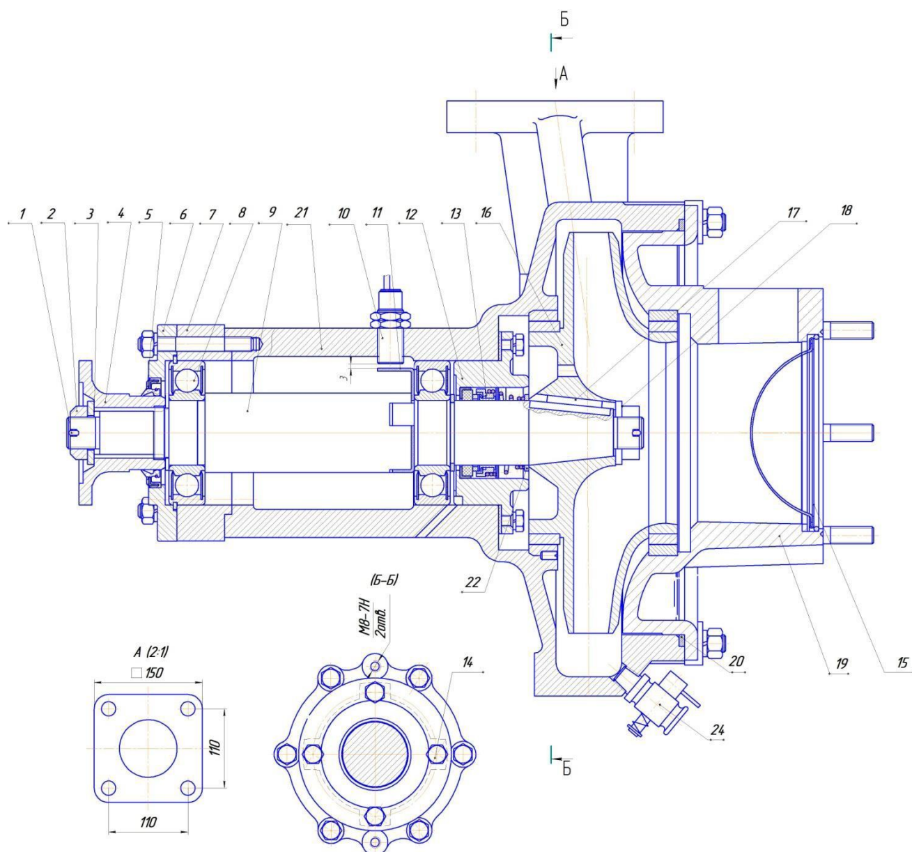
Рис. 2 Насос
