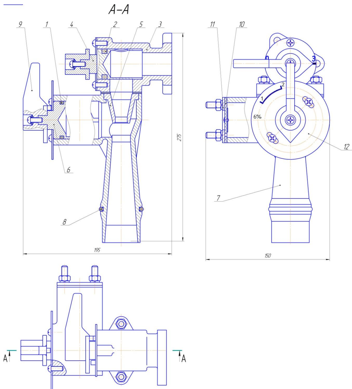
Рис. 6 Пеносмеситель ПС-2
