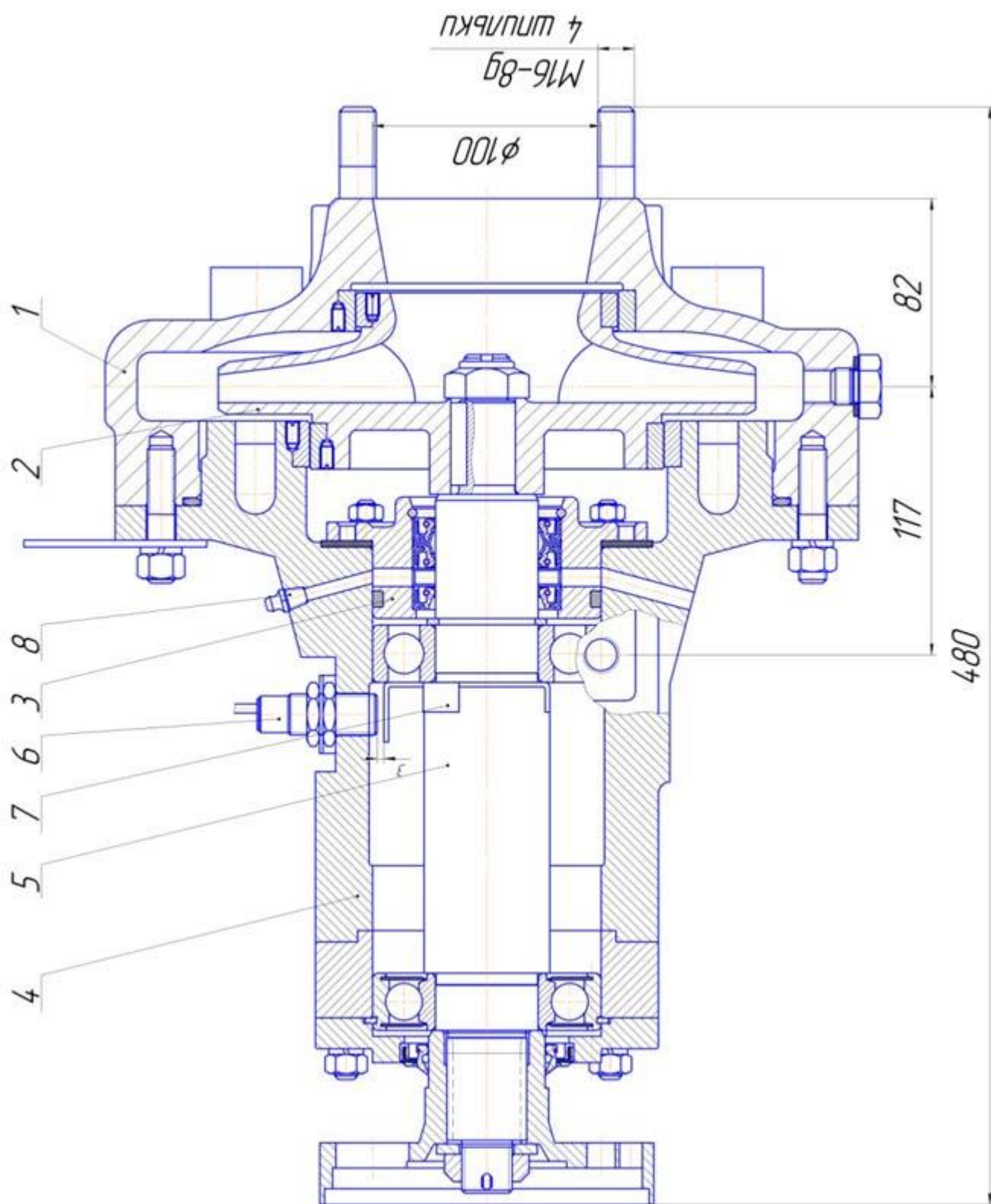
Рис. 4 Насос
